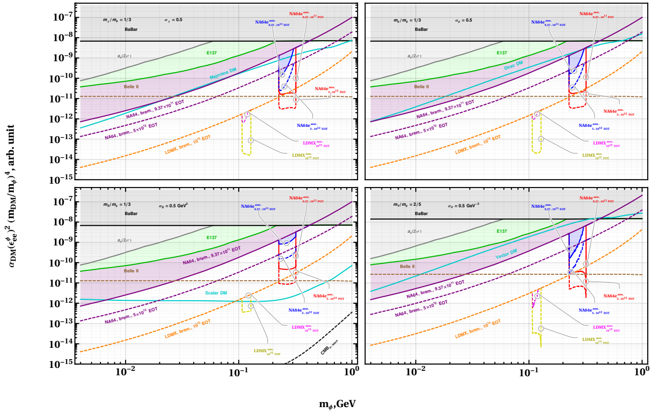
Рисунок 3.6 — Ограничения на константу взаимодействия скалярного медиатора с электроном как функция его массы из реакций рождения медиатора на ядре и в резонансном процессе для невидимой моды на основе отсутствия сигнала в экспериментах с фиксированной мишенью (раздел 3.1.1). Черной непрерывной линией показаны ограничение на основе эксперимента ВаБар [205]. Зеленой непрерывной линией показаны ограничения из эксперимента E137 [21; 199; 201]. Пунктирной коричневой линией показаны пределы из планируемых результатов эксперимента Belle II [21]. Исключение из СМВ для скалярной темной материи показаны пунктирной черной линией [12]. Фиолетовой и оранжевой непрерывной (пунктирной) линиями показаны текущие (планируемые) ограничения для экспериментов NA64e и LDMX, соответственно. Красной и синей (желтой и розовой) линиями показаны ограничение из резонансной реакции для позитронной и электронной мод из эксперимента NA64e (LDMX), соответственно, где для текущей статистики используется непрерывная линия, а планируемая показана пунктирной. Реликтовые кривые для соответствующего типа темной материи изображены бирюзовой линией. Соответствие панели и типу темной материи представлено как: левая верхняя - майорановская, левая нижняя - скалярная, правая верхняя - дираковская и правая нижняя - векторная.
