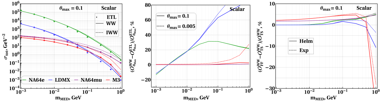
Рисунок 3.3 — Общее . На приведенном рисунке показано полное сечение и его относительная разница в случае различных углов вылета медиатора и моделей атомных форм-факторов, где цветом обозначены эксперименты NA64e (зеленый) LDMX (синий) NA64 \mu (фиолетовый) и M 3 (красный). Первая фигура . Полное сечение излучения скалярного медиатора на ядре в зависимости от массы с использованием приближения Вайцеккера-Вильямса (непрерывная линия), приближения улучшенного Вайцеккера-Вильямса (пунктирная линия) и расчетов на уровне дерева (точки). Константа взаимодействия для скаляра и лептона принимает следующее выражение c_{ll}^S = 1 . Вторая фигура . Относительная разница полных сечений в подходе Вайцеккера-Вильямса и расчетов на древесном уровне в случае различных максимальных углов вылета \theta_{\max} = 0.1 и \theta_{\max} = 0.005 . Третья фигура . Относительная разница полных сечений сечений для хельмовского (непрерывная линия) и экспоненциального (пунктирная линия) форм-факторов, где за эталонный взят форм-фактор Тсаи-Шиффа.
