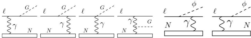
Рисунок 2.1 — Диаграммы процессов излучения скалярного \phi и тензорного G медиаторов на ядре N при падении на ядро лептона l .
