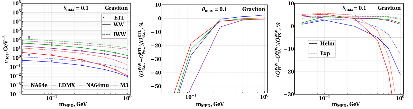
Рисунок 3.4 — Описание графика аналогично 3.3, где соответствующая константа взаимодействия для тензорного медиатора принимает следующие выражение c_{ll}^G = 1 \text{ ГэВ}^{-1} .
