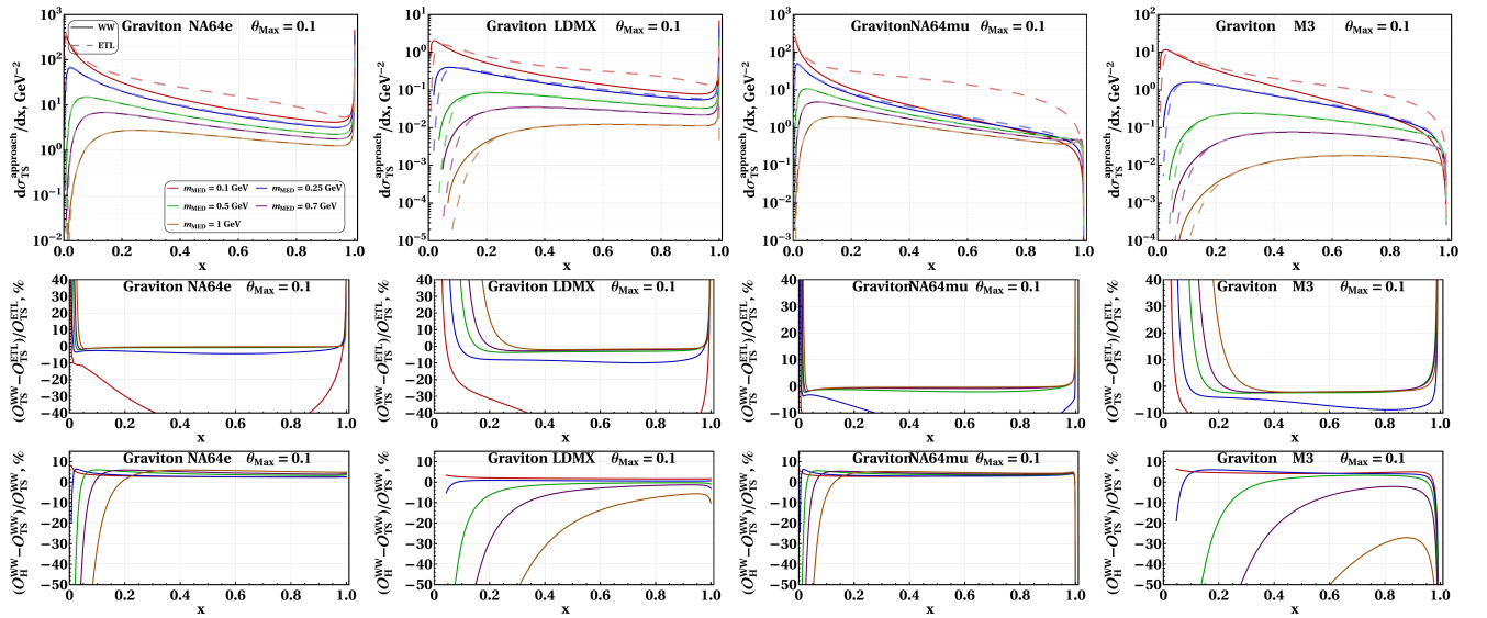
Рисунок 3.2 — Описание графика аналогично 3.1, где соответствующая константа взаимодействия для тензорного медиатора принимает следующие выражение c_{II}^G = 1 ГэВ
